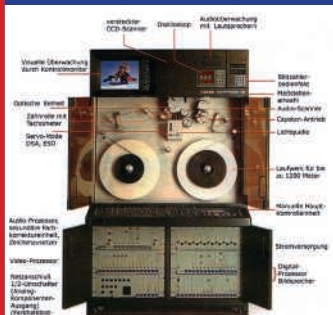
DIGITALER FILMABTASTER SDL-1001
