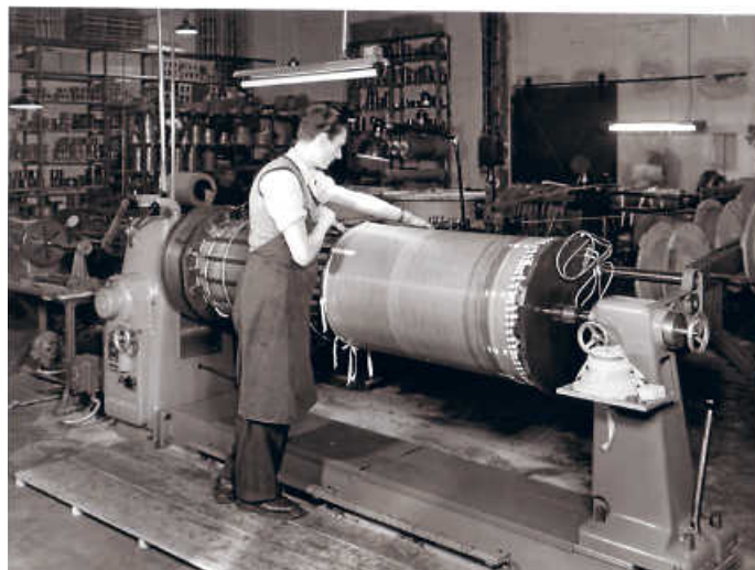
Fertigung einer Trafospule an der Drehbank/ Berlin Reinickendorf Foto: G. Gritschke
