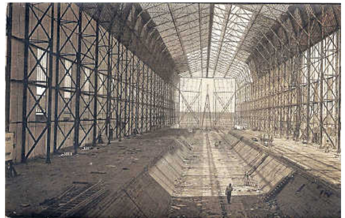
Ein seltener Blick in das Innere der fast leergeräumten Halle in Richtung Tor und Fluggelände. Die wenigen Arbeiter verlieren sich im Lauf- und Wartungsgraben der Halle. Die Aufnahme gibt Details der Hallenkonstruktion detailliert frei Foto: HBV
